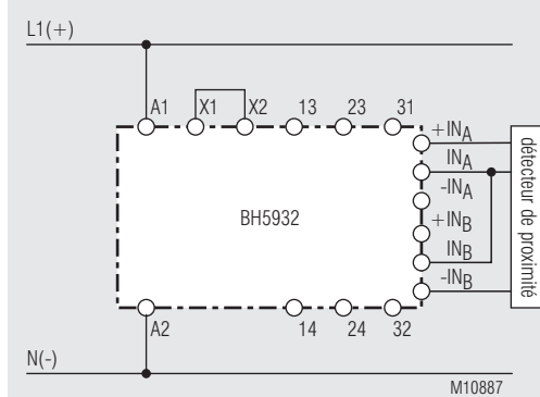
Branchement détecteur de proximité; convient jusqu'à SIL2, Performance Level c, Cat. 2 (Une condition primordiale pour le maintien de la catégorie 2 est le contrôle à intervalles réguliers de la fonction de sécurité).
