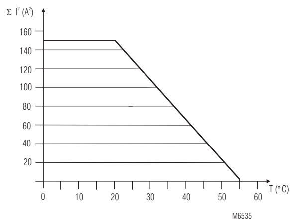
Courbe limite d'arc (contacts temporisé)
